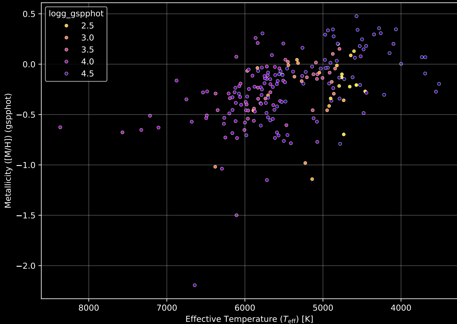
APOGEE DR17 Field: [K2_C12_082-60_btx] Stellar Population Parameters (n= 207)
